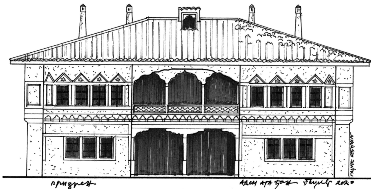
9. Палата Адем аге Ђона, цртеж главне фасаде
