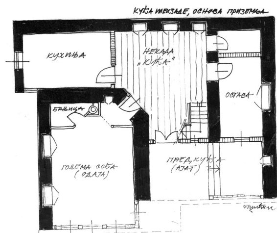
5. Призрен, палата Шехзаде, цртеж основе и изглед фасаде
